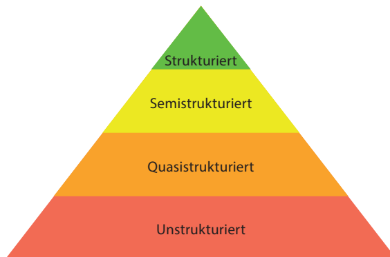
Abb. 1–2 Datenpyramide
